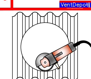
1. Realizar el corte en la lámina se Asbesto con Cortadora de Disco.
