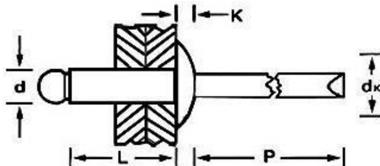
Dimensiones en milésimas de pulgada
